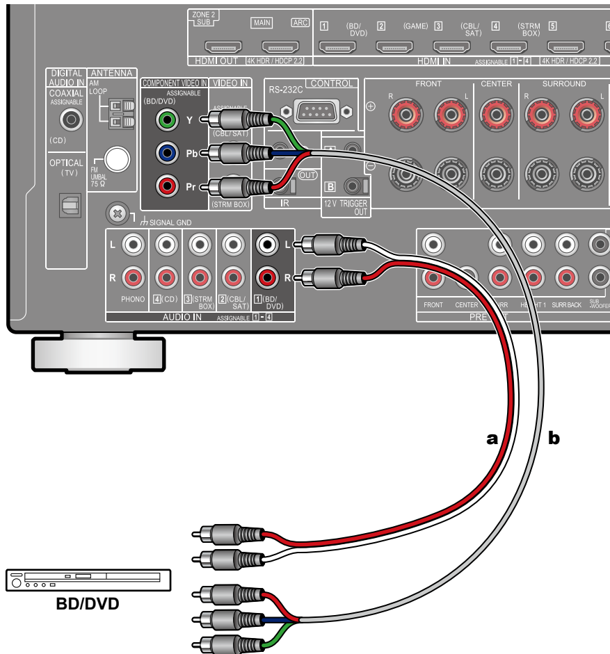
a Câble audio analogique, b Câble vidéo composante
