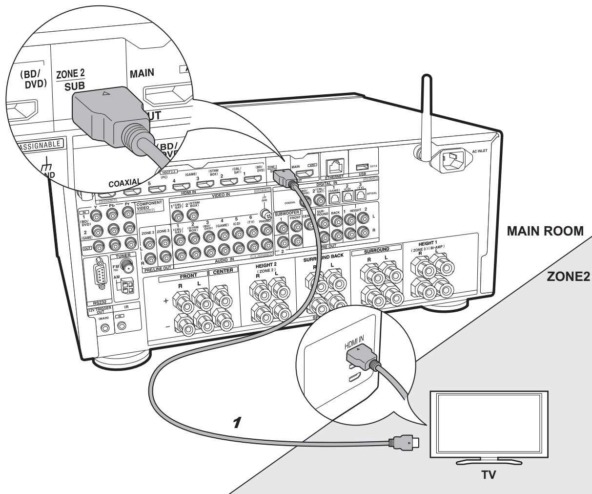
1 Cable HDMI
