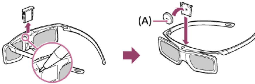
(A) CR2025 Côté (-)
