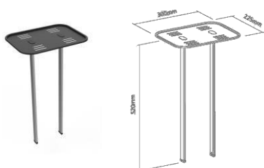
Étagère caméra Réf. 030-5093
