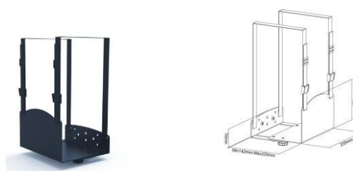
Support unité centrale Réf. 030-5094
