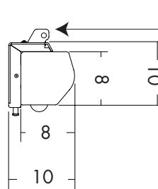
Côté du carter avec patte de fixation
