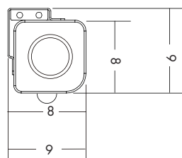
Côté du carter avec patte de fixation
