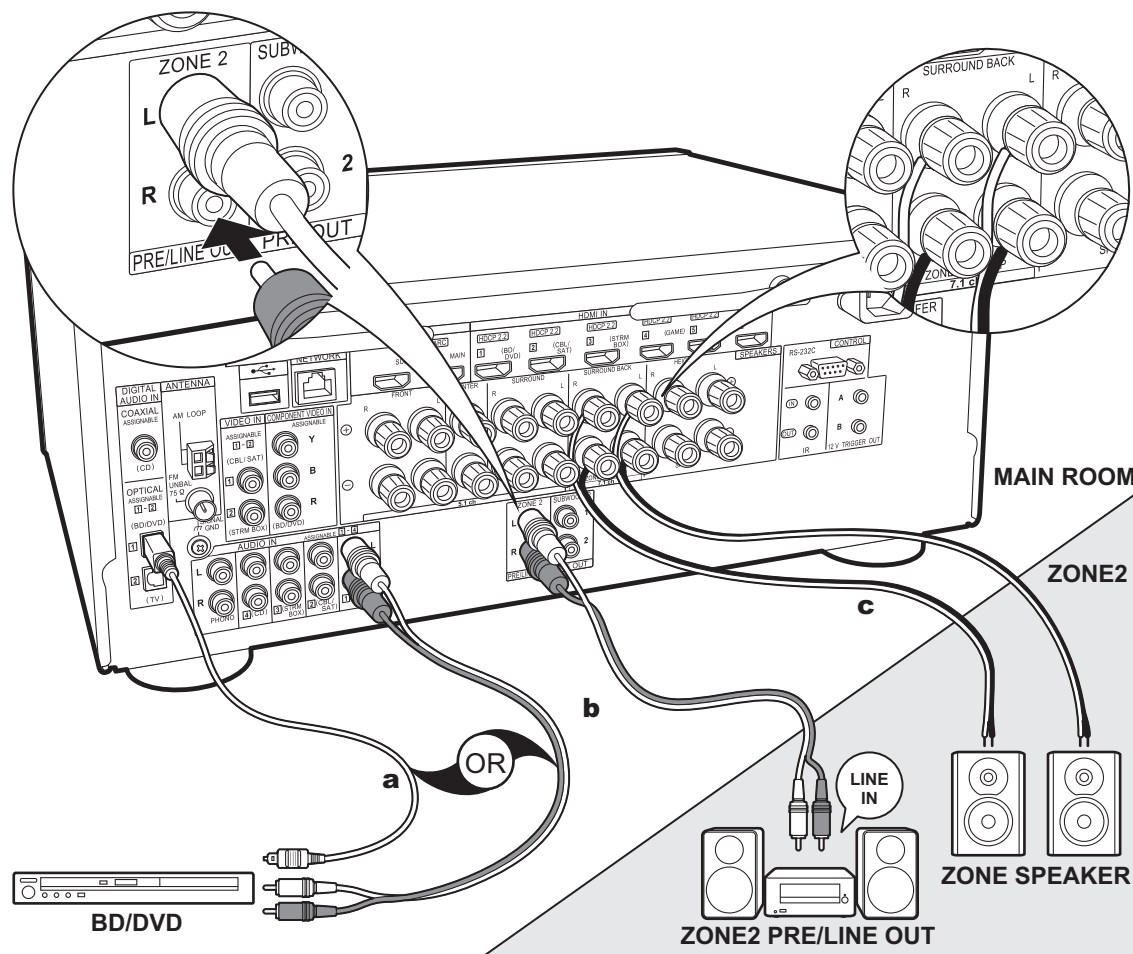
a Cable óptico digital, b Cable de audio analógico, c Cable de altavoz
