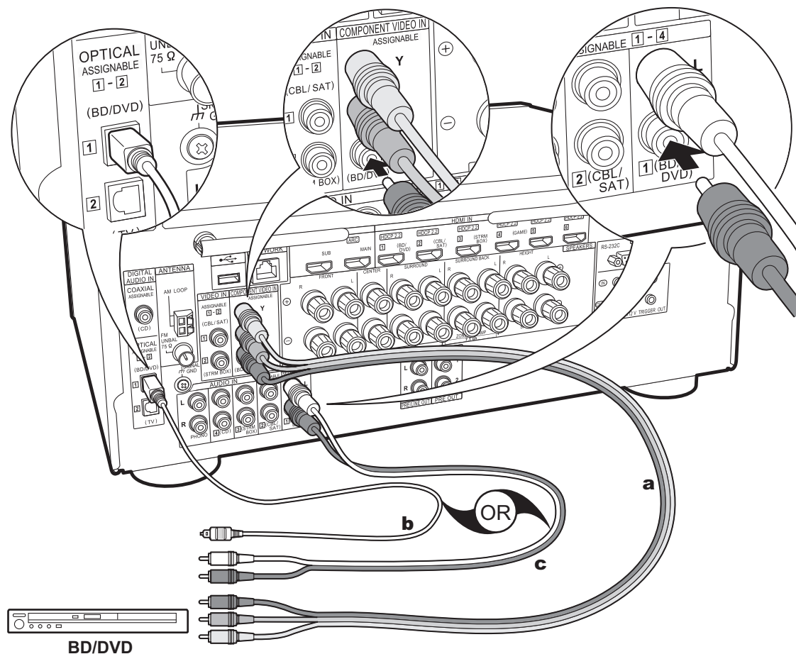
a Cable de vídeo componente, b Cable óptico digital, c Cable de audio analógico
