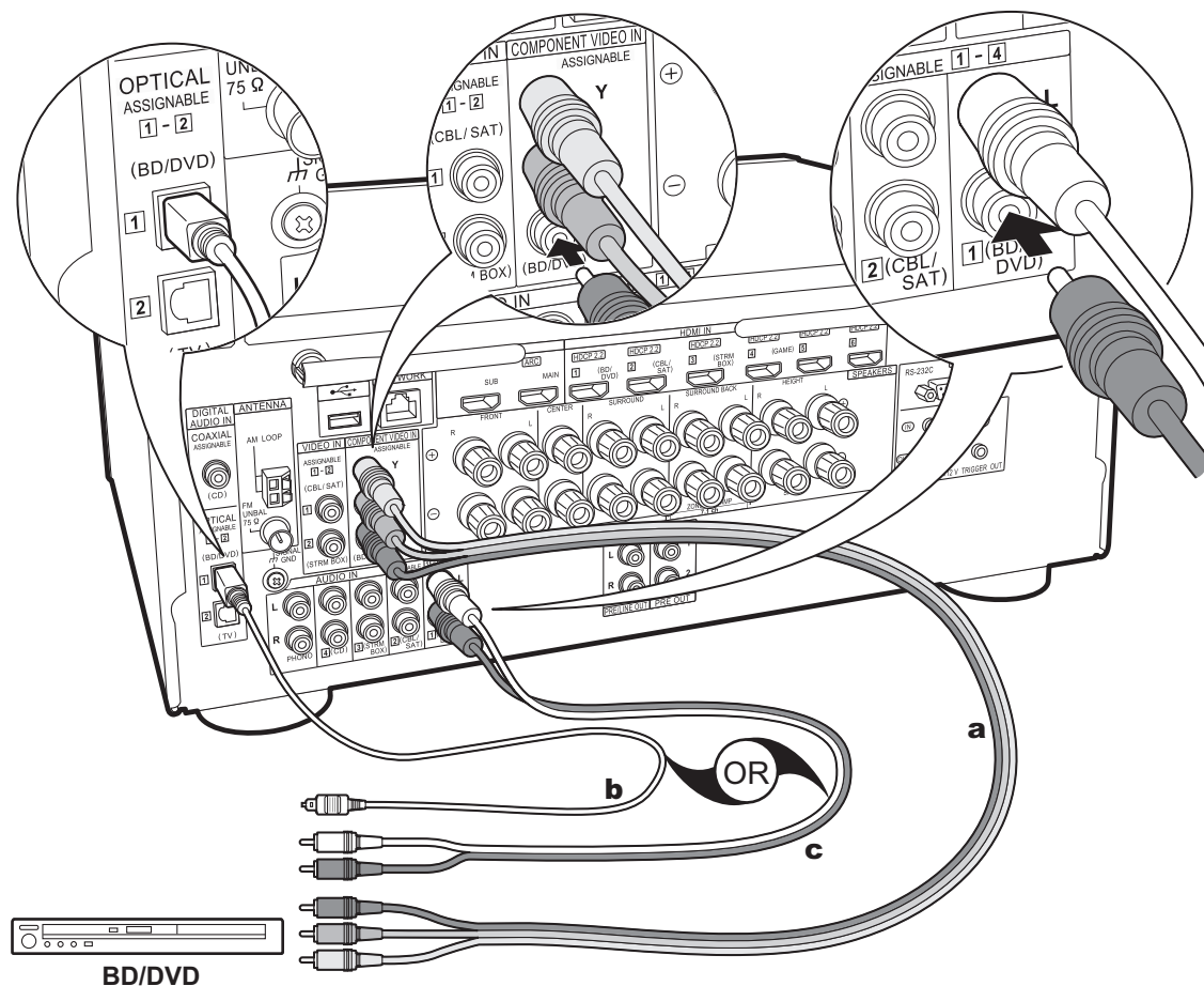
a Câble vidéo composite, b Câble optonumérique, c Câble audio analogique
