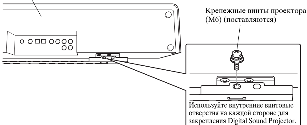
Digital Sound Projector Вид снизу
