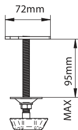
GROMMET CLAMP
